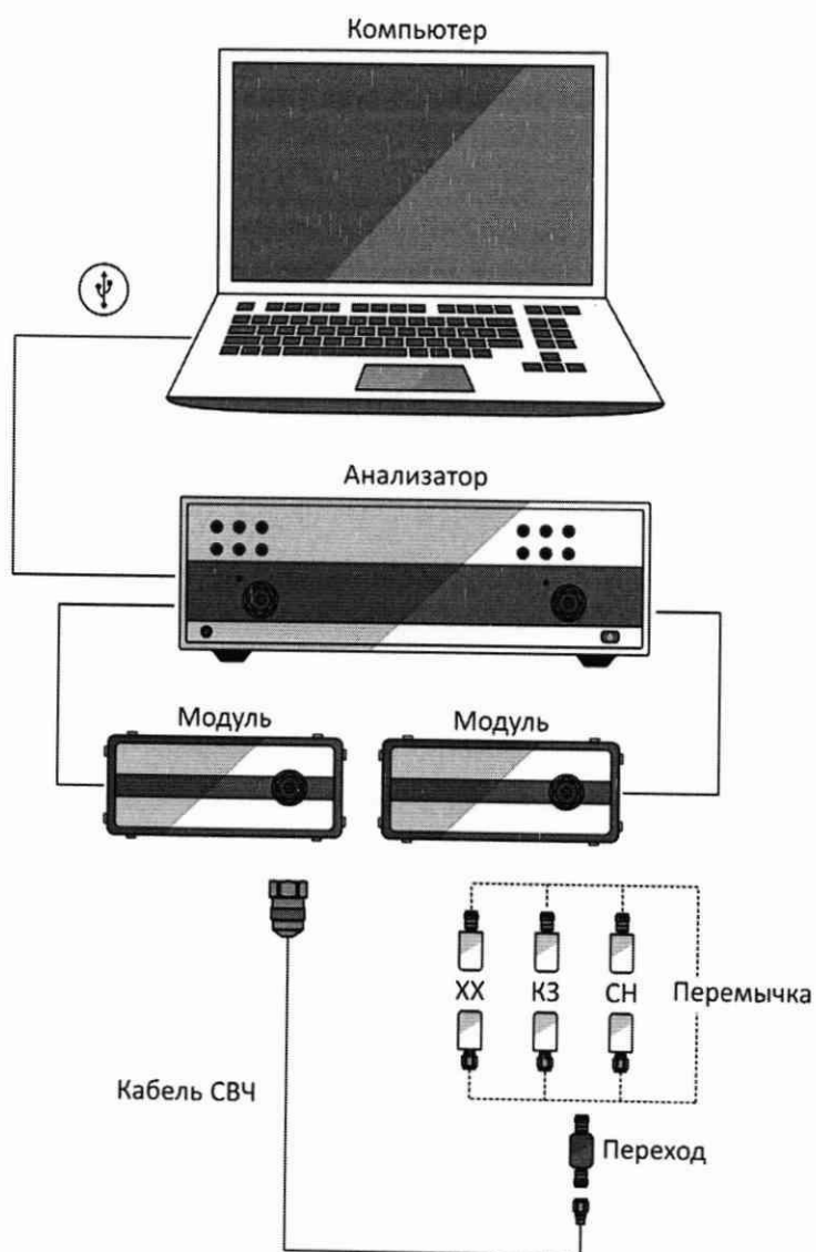
Рисунок А.11 – Схема измерений (проведение полной двухпортовой «калибровки»)
