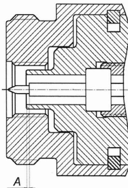
Рисунок А.2 – Присоединительный размер А
