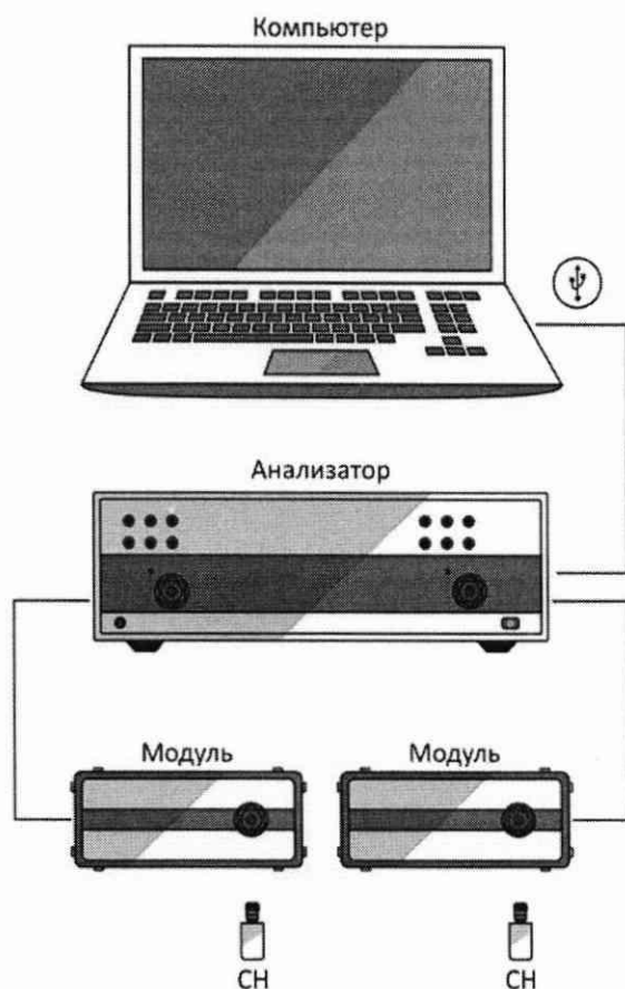
Рисунок А.6 – Схема измерений
